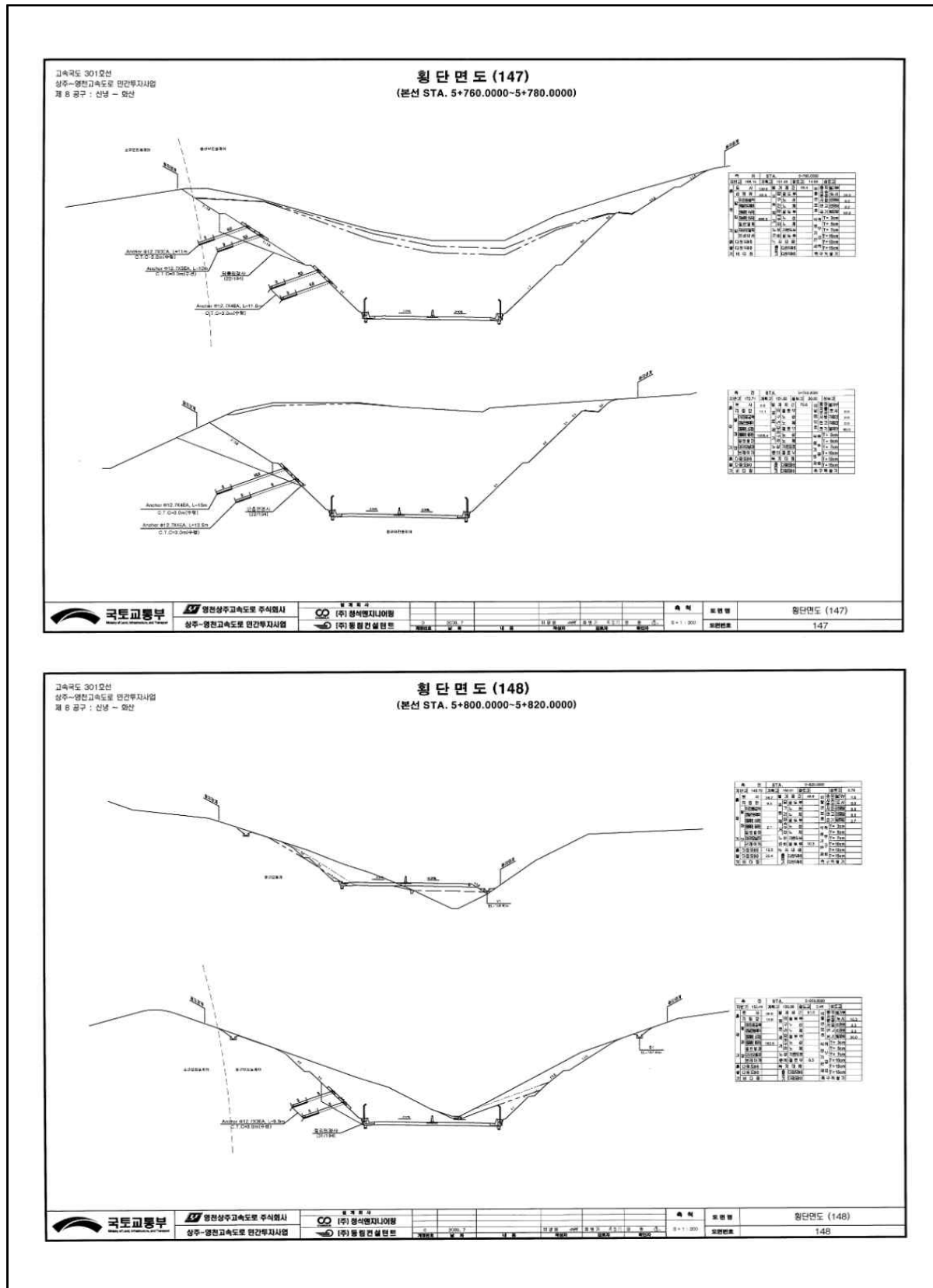
[그림 49.4] 표준횡단면도
