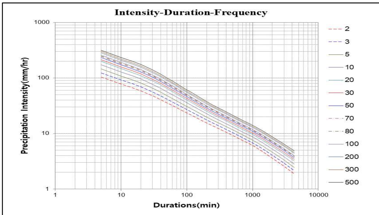
【그림 49.9】 영천지역 IDF곡선
