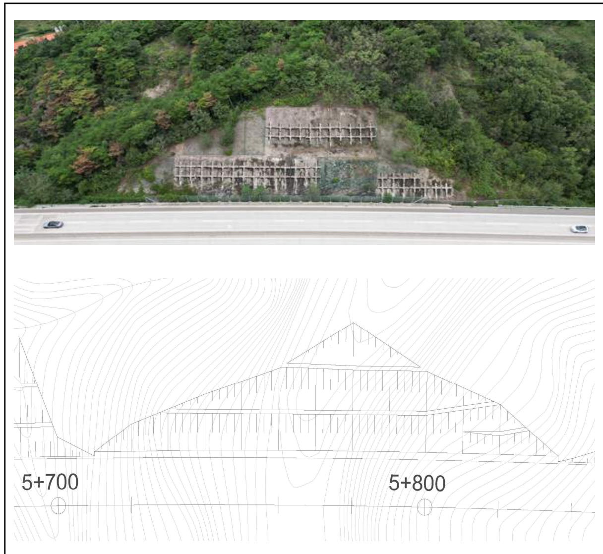
【그림 49.14】 상주절토49 검토대상 비탈면구간
