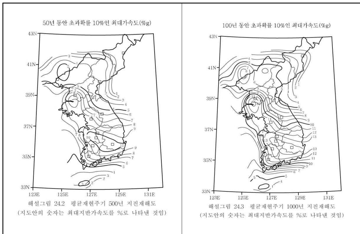
【그림 49.12】 평균재현주기 500년 및 1000년 지진재해도
